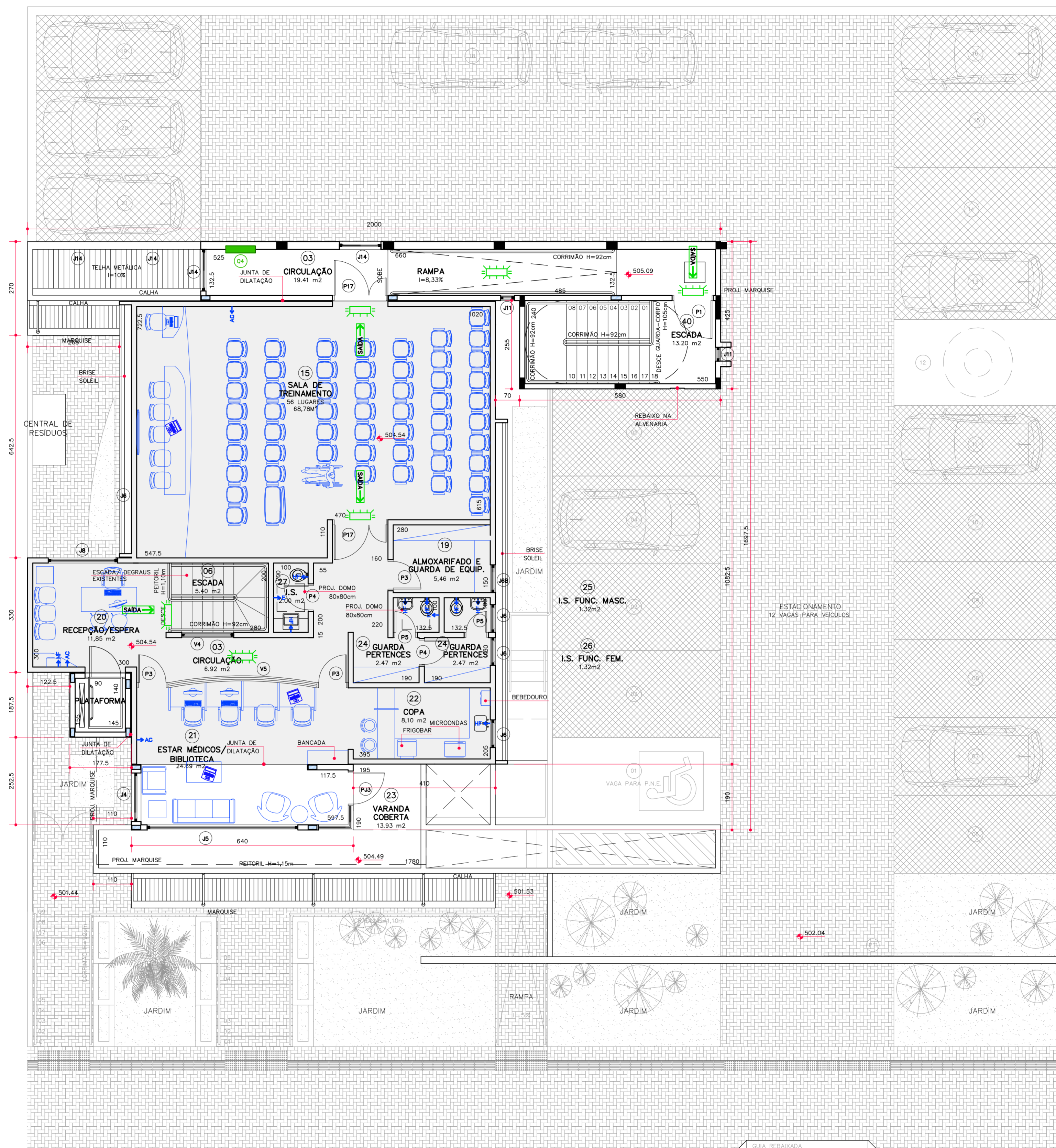
PLANTA PAV. SUPERIOR - LAYOUT ESC. 1:75
